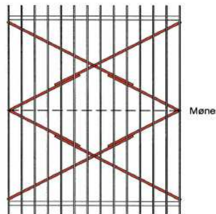
Ved brede, korte bygg kryssavstives hver takflate!
