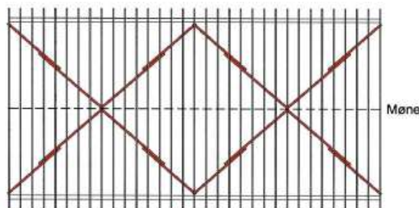
Ved lange bygg gjentas avstivningen!
