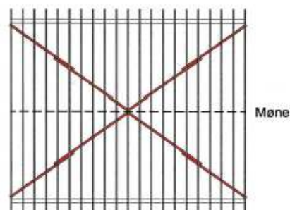
Avstivningen monteres fra gavlvegg (ved raft) mot mønet!
